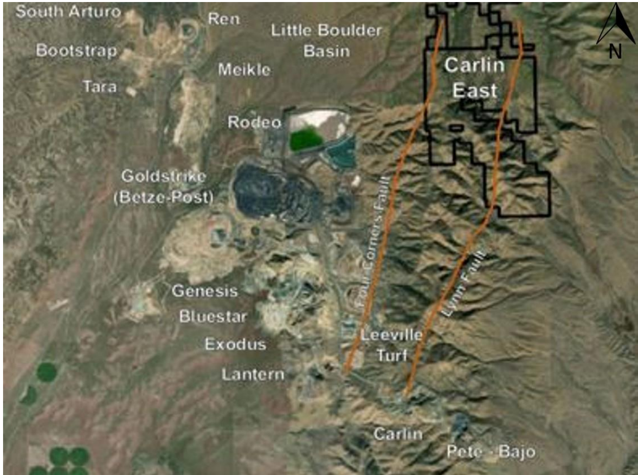
Figure 1 : Localisation du projet Carlin-East de Ridgeline Minerals-couloir minéralisé Carlin
